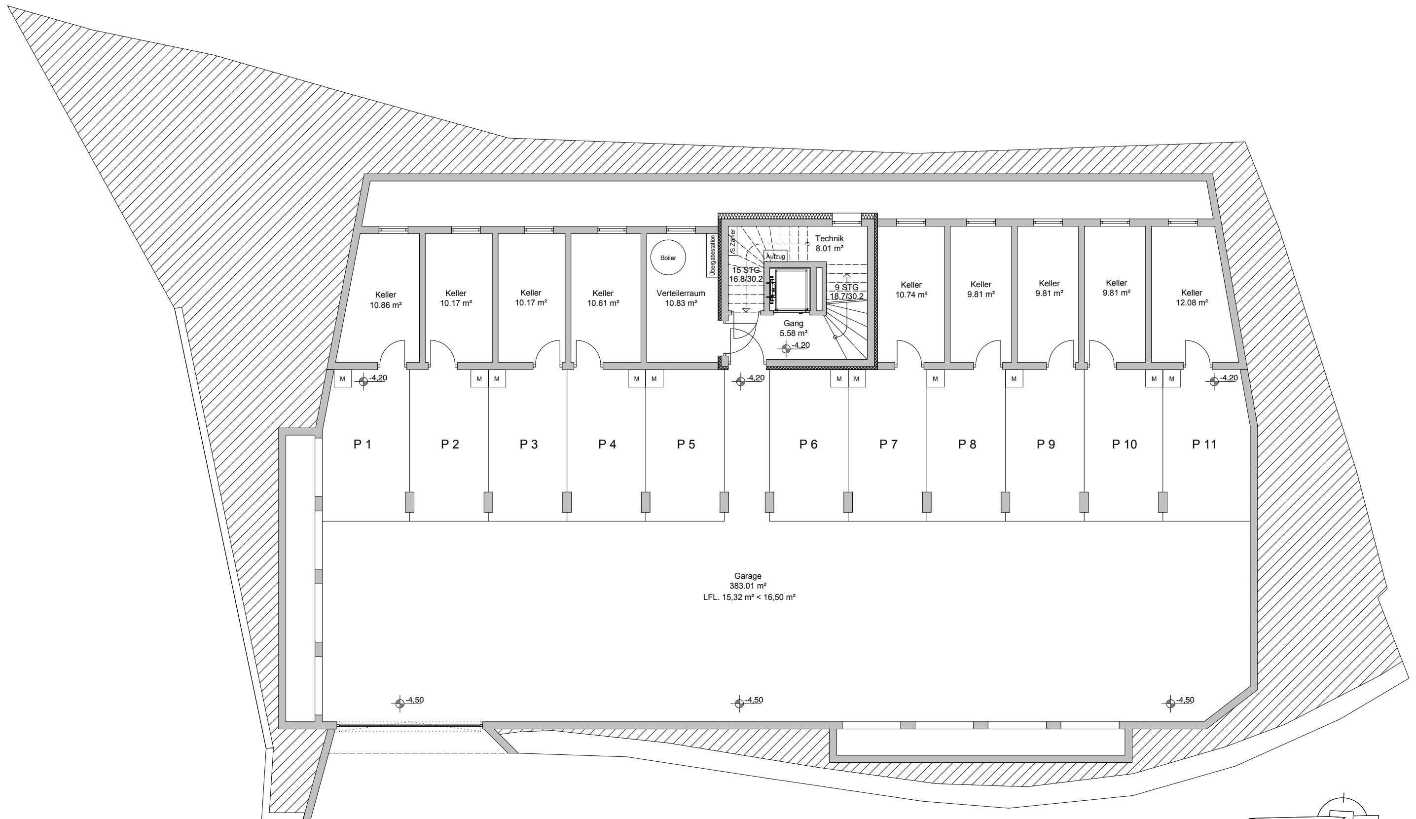
Kellergeschoss
